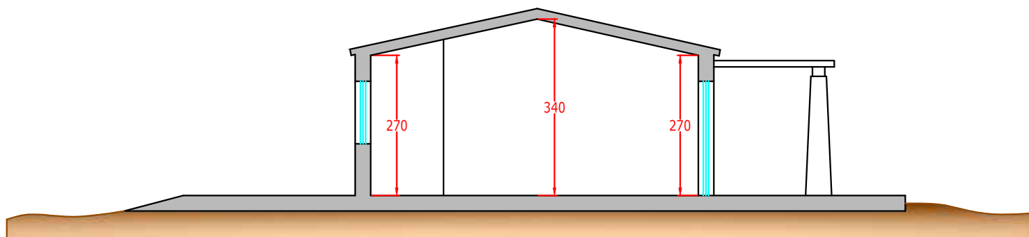
SEZIONE TIPO
